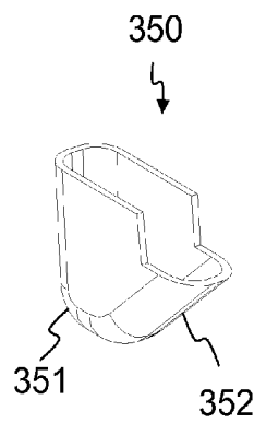
FIG. 5E
