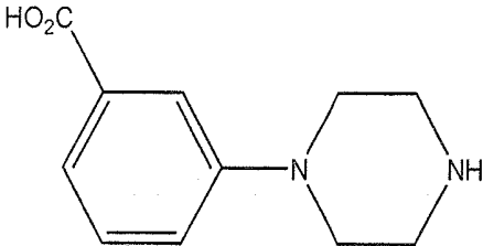
Hapten - A
