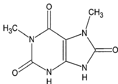
1,7-DMU (1,7-dimethyluracil)
