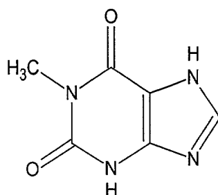
1X (1-methylxanthine)
