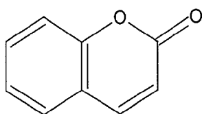
Coumarin
