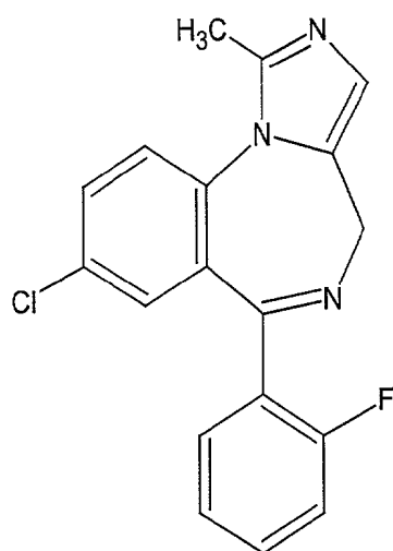
MDZ (Midazolam)
