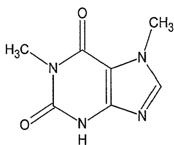
1,7-DMX (1,7-dimethylxanthine)
