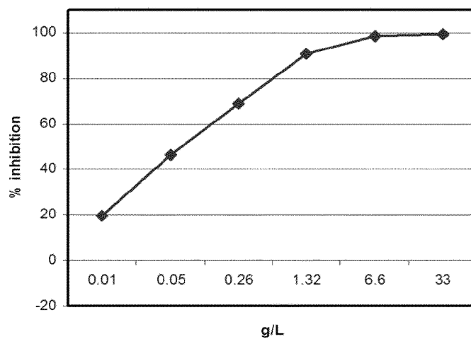
FIG. 8C CAP-e assay
