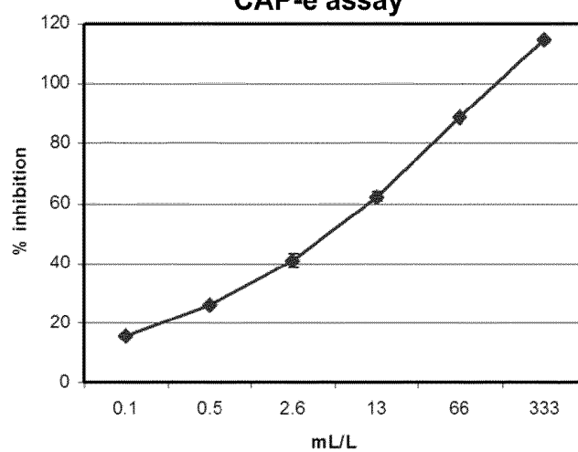
FIG. 9C CAP-e assay
