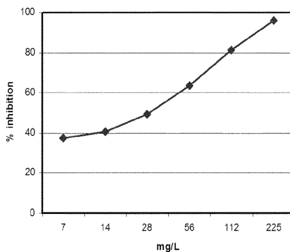
FIG. 7C CAP-e assay
