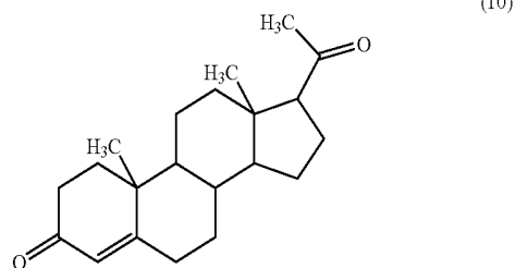
Progesterone
