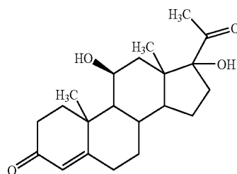
Cortisol
