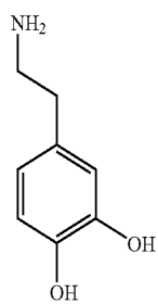
Dopamine
