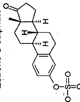
Estrone-3-sulphate
