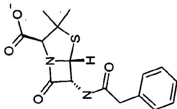
Benzylpenicillin
