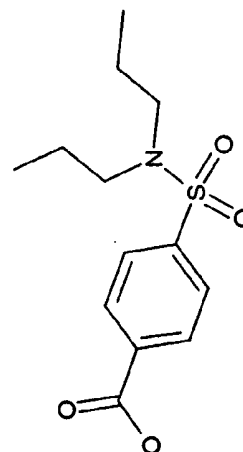
Probenecid
