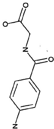
Para-amino-hippurate
