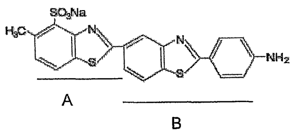
Primulin
