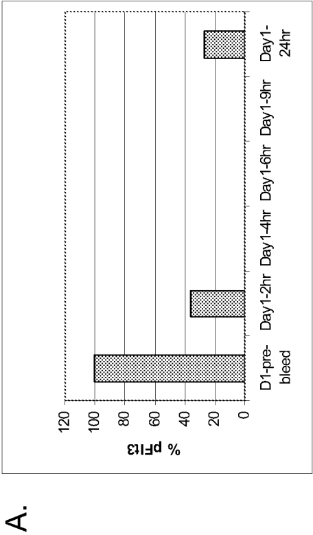
pFlt3/tFlt3 trend
