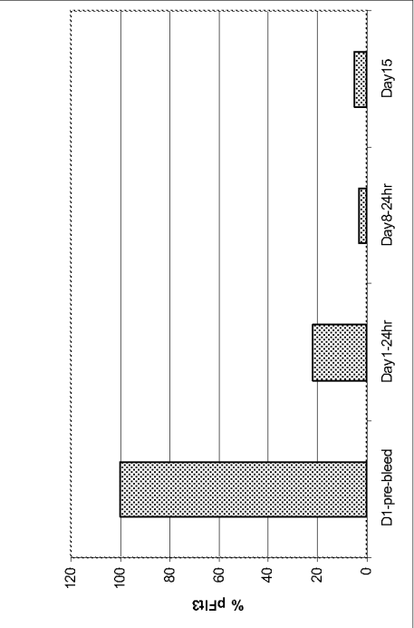
pFlt3/tFlt3 trend
