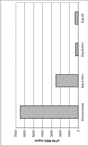
pFlt3
