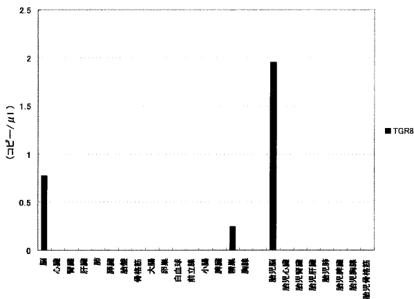
Multiple Tissue Panel 1μlあたりのTGR8のコピー数
