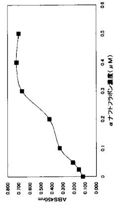
αナフトフラボンのドーズ レスポンスカーブ(CYP19 133I)
