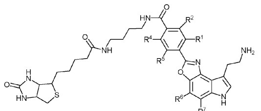
セロトニン(5-HT)類似体Ia
