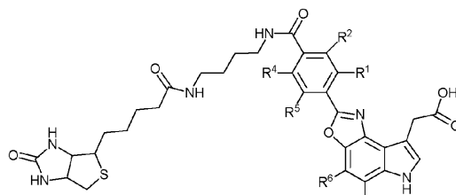
5-ヒドロキシインドール酢酸(5-HIAA)類似体Ib
