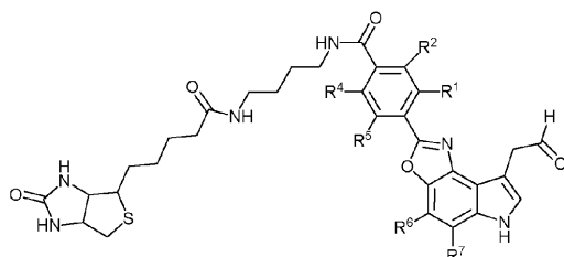
5-ヒドロキシインドールアセトアルデヒド類似体Ic
