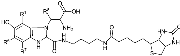
5-ヒドロキシトリプトファン(5-HTP)ピオチン誘導体 Ila
