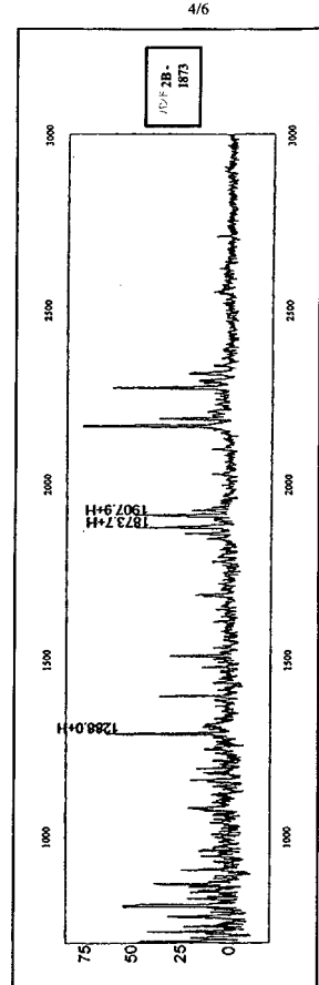
FIGURE 4 バンド2Bのトリプシン消化 Seidi-TOF スペクトル
