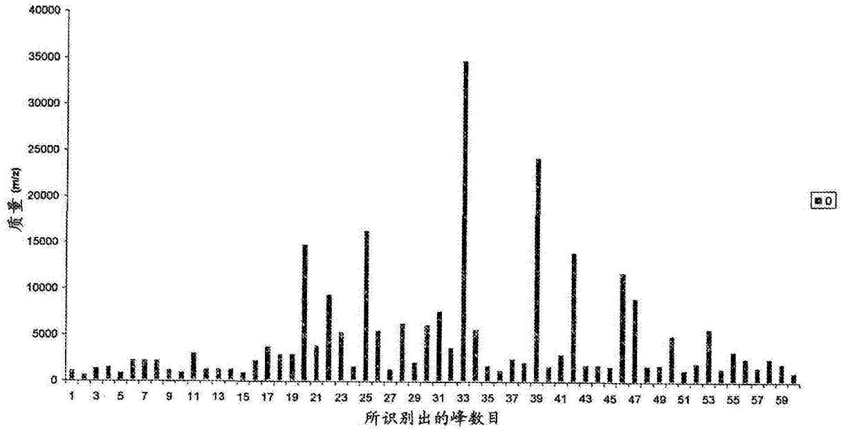
经MGO修饰的MRJPI的胰蛋白酶消化物的MS分析
