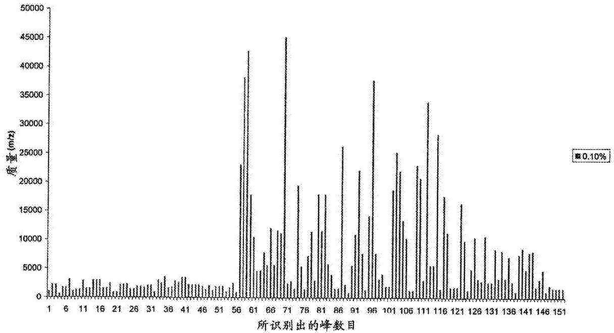
经MGO修饰的MRJPI的胰蛋白酶消化物的MS分析
