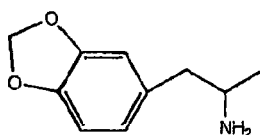
3 MDA
