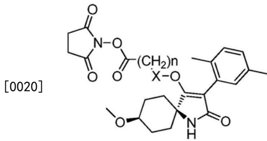
式 E 结构式
