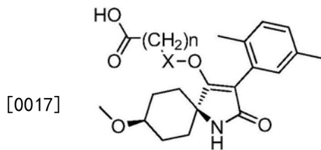
式 D 结构式
