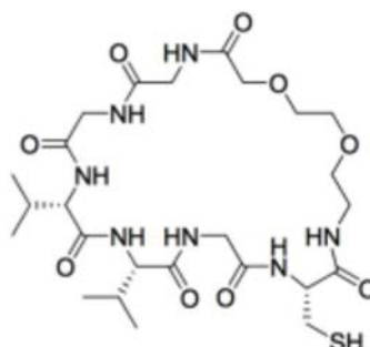
环状(C-PEG2-GGVVG)
