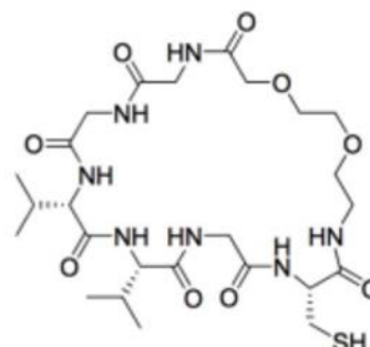
环状 (C-PEG2-GGVVG)
