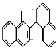
苯并[a]荧蒽
