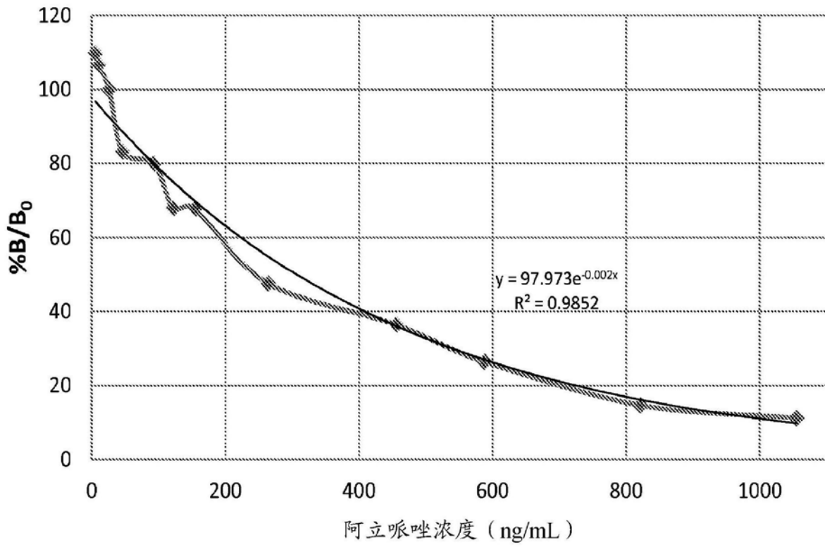
阿立哌唑校准曲线-- GC/MS 高于MM1的MM浓度值 %B/B 0 对阿立哌唑浓度
