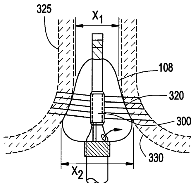
FIG. 3E PRIOR ART
