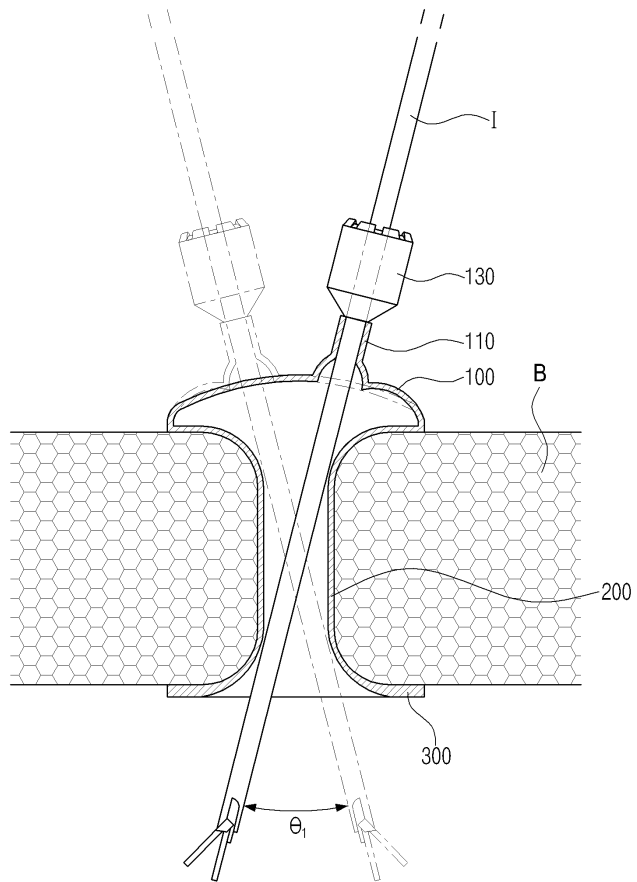
도면4
