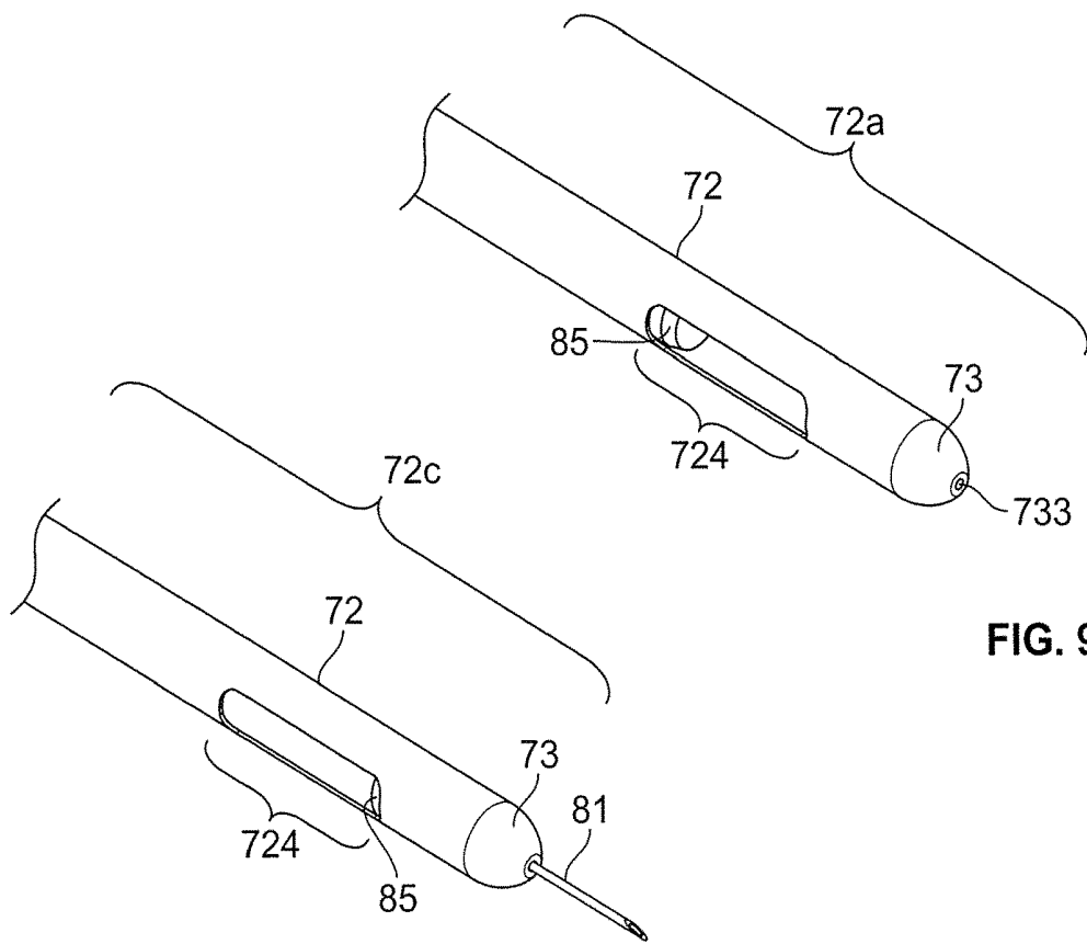
FIG. 9D
