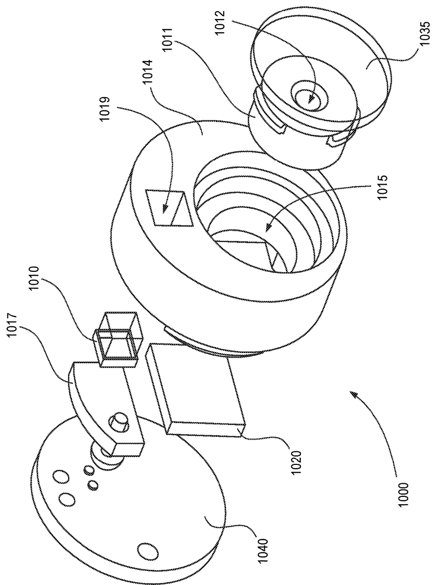
FIG. 10B
