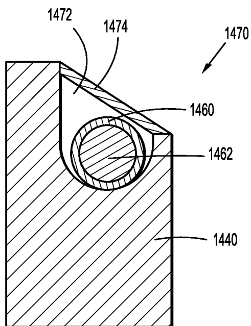
X-X FIG. 16
