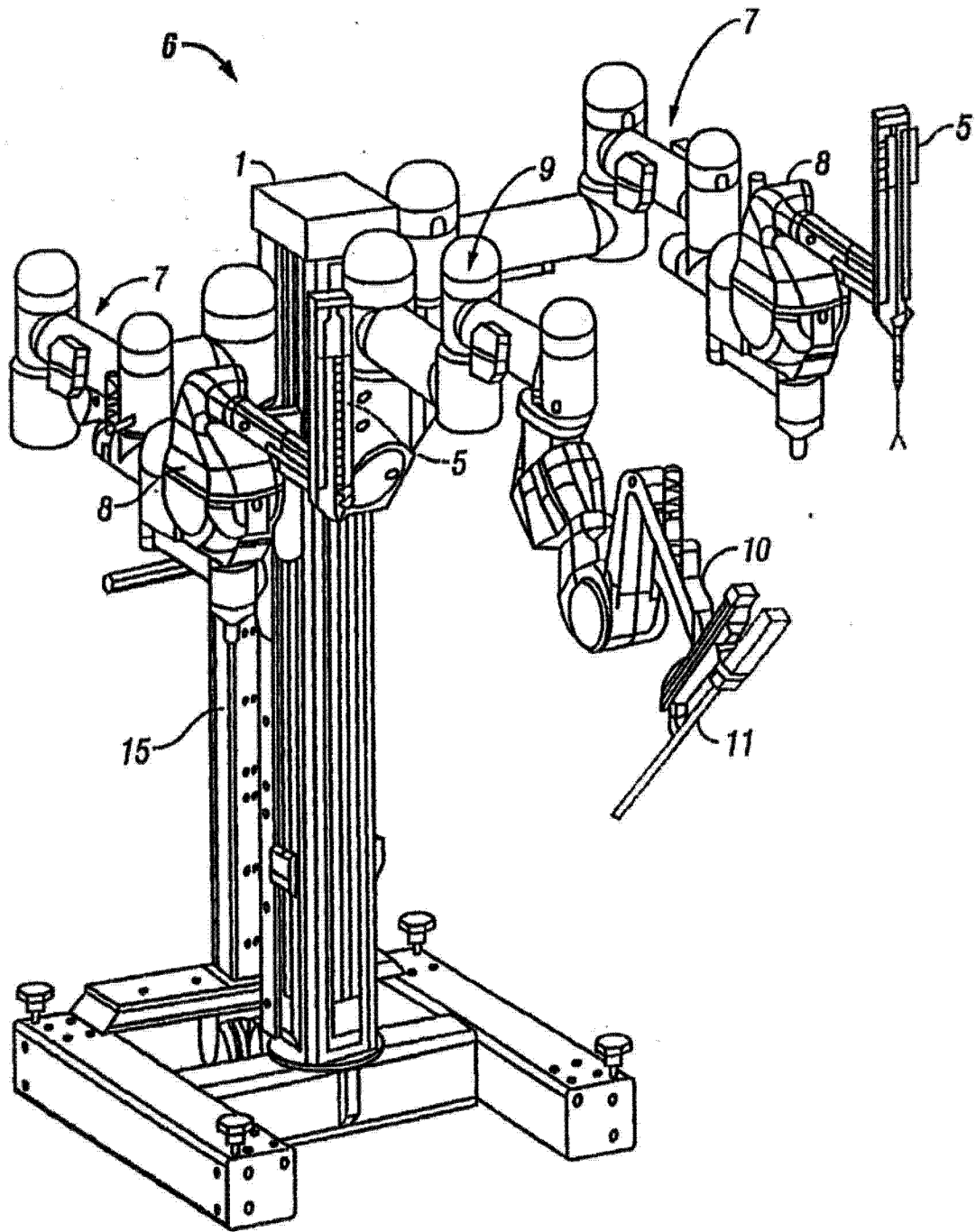
图 2(现有技术)
