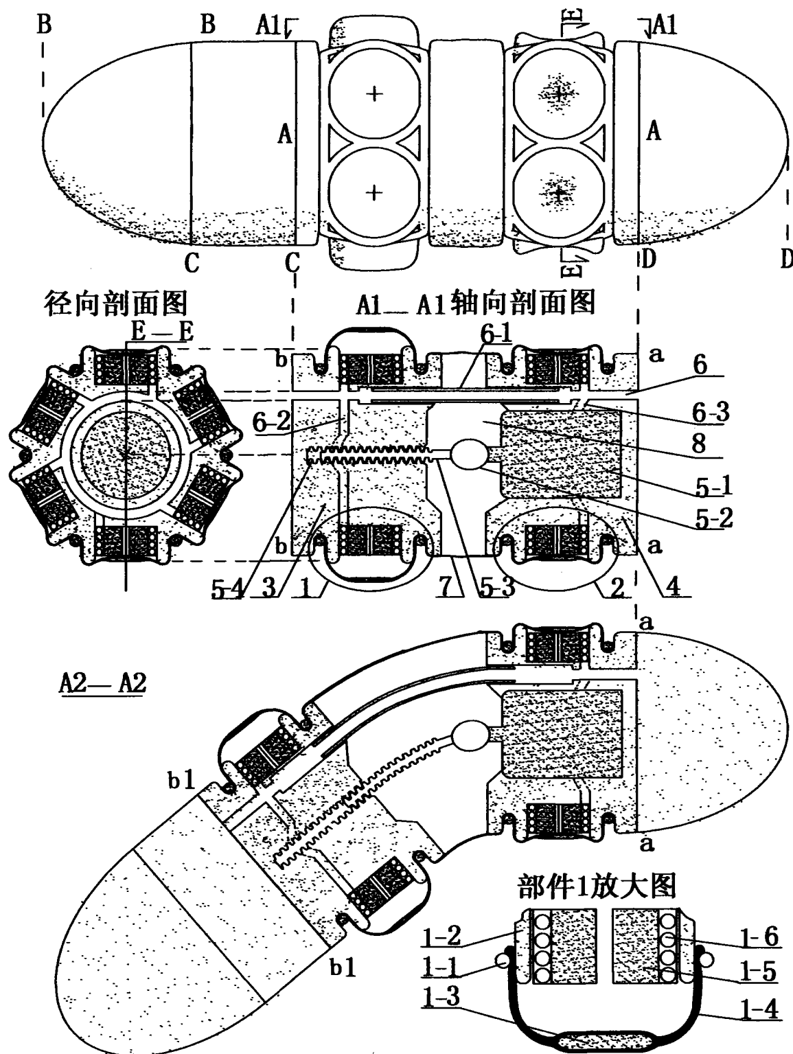
比例约 2:1 遥控式纯电力肠镜外形示意图
