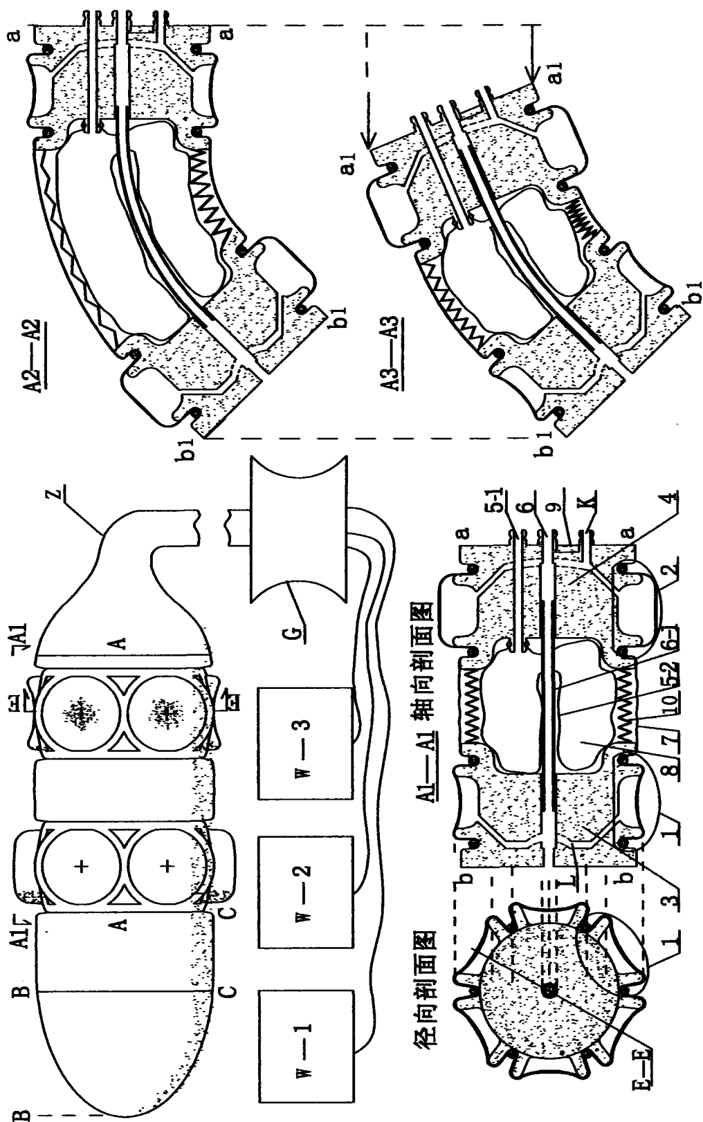
比例约 2:1 分体式流体动力肠镜外形图
