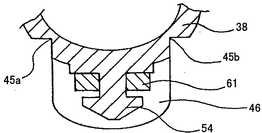
R-R' 剖面
