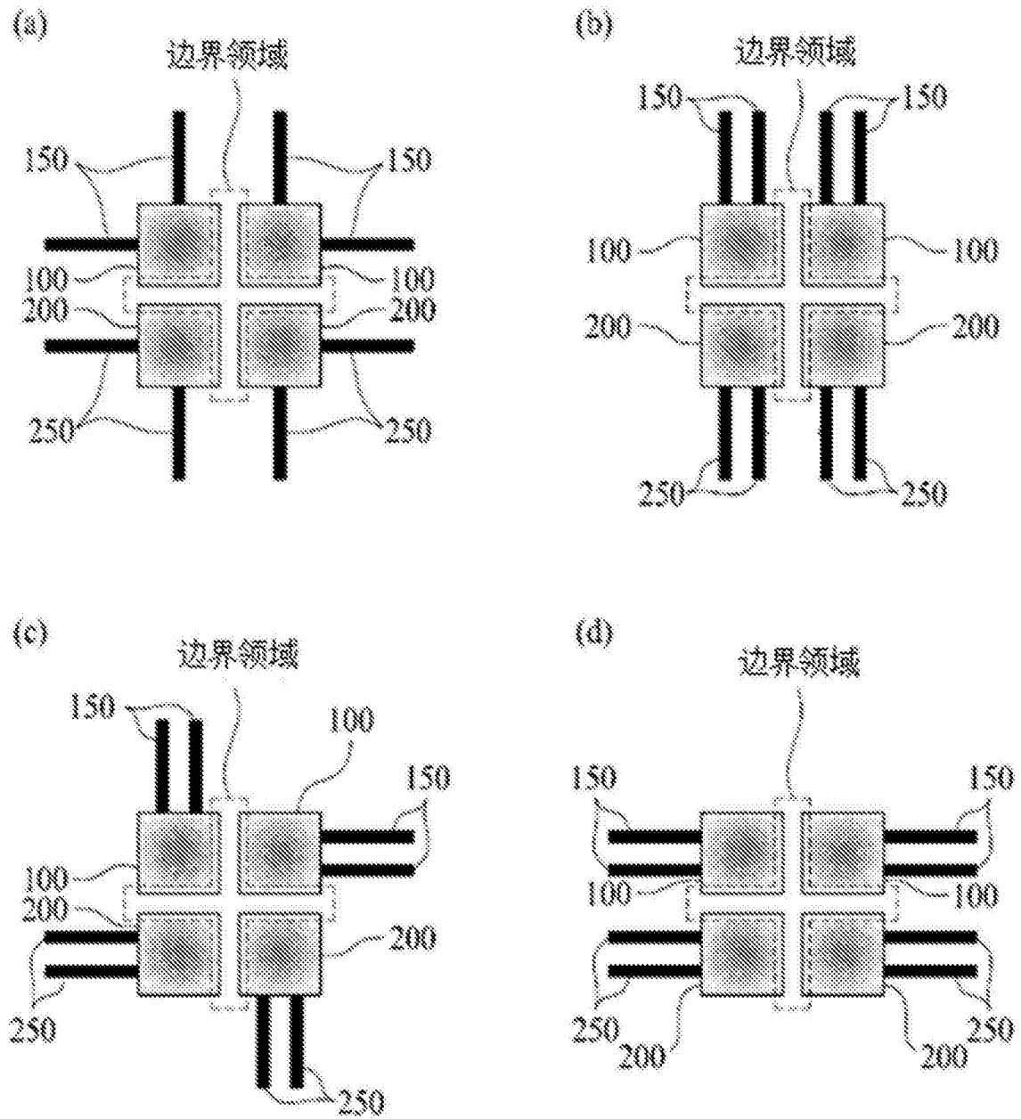
图16
