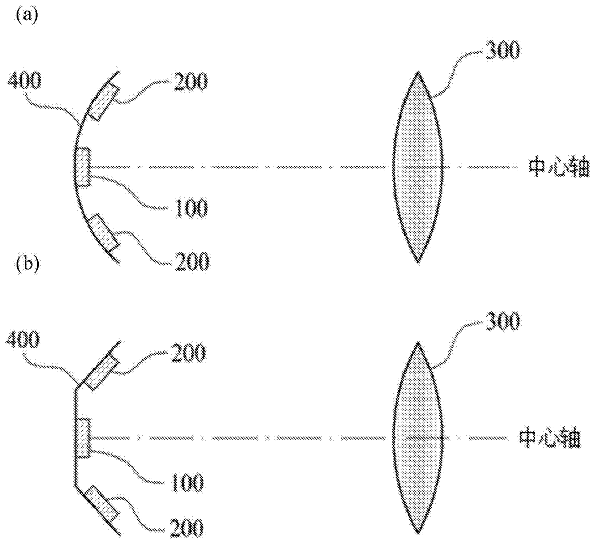
图13
