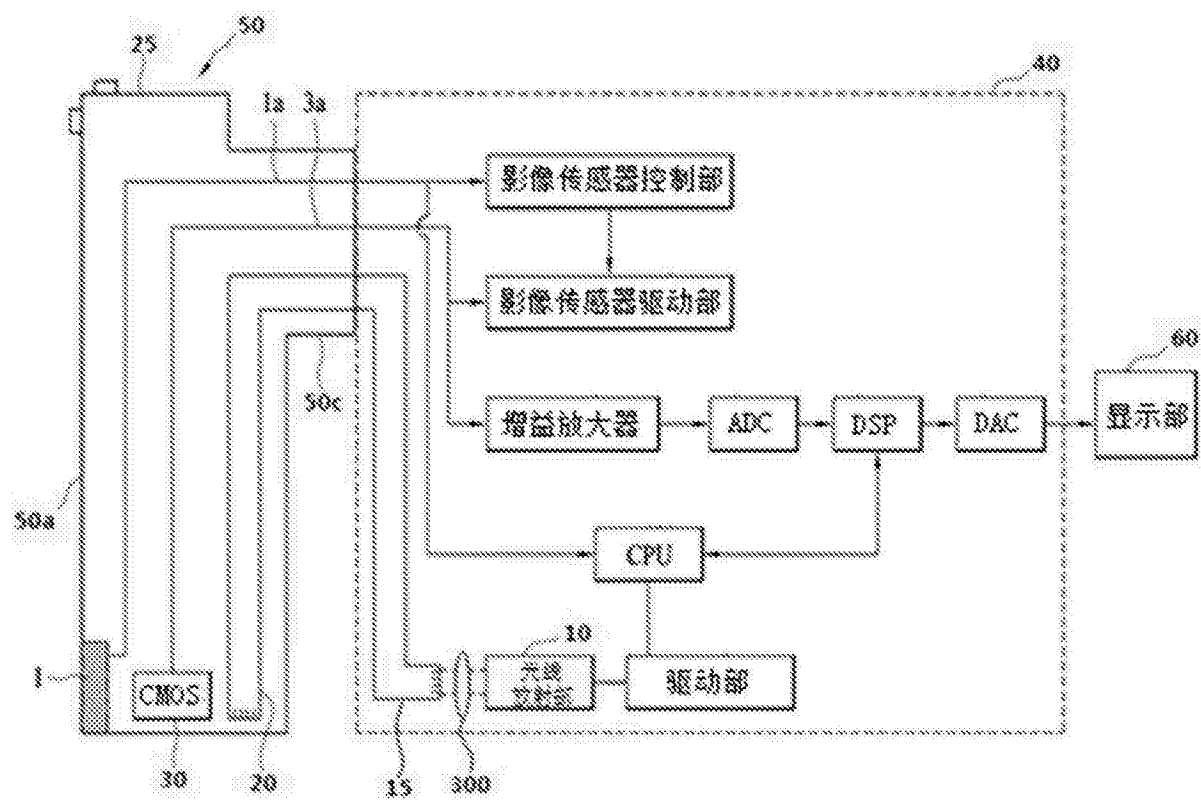
图 20
