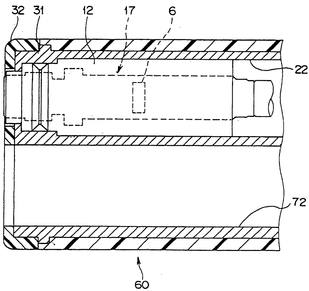
III-III 截面
