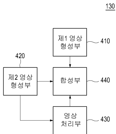
도면5
