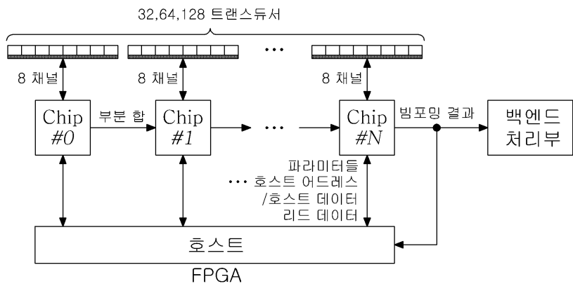
도면8
