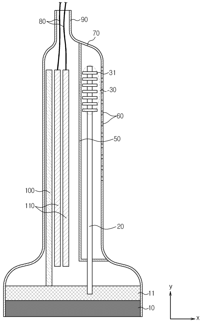
도면3
