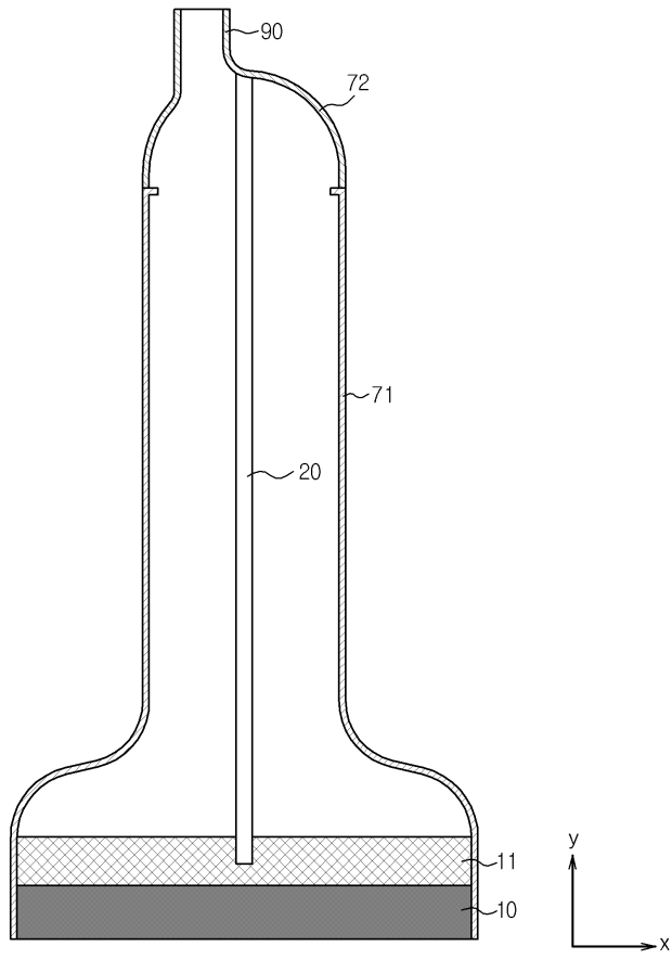
도면10
