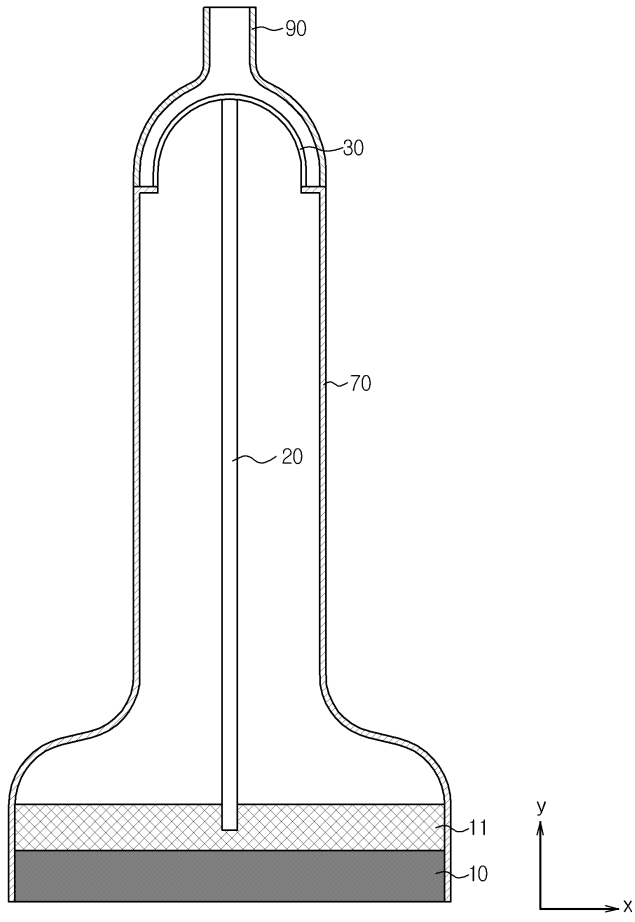
도면8
