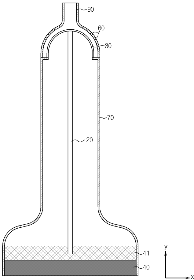
도면7
