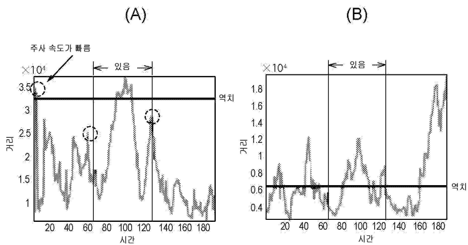
도면15
