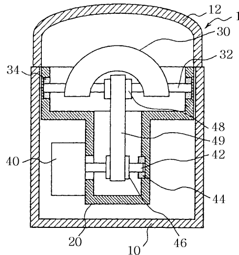
도면1b
