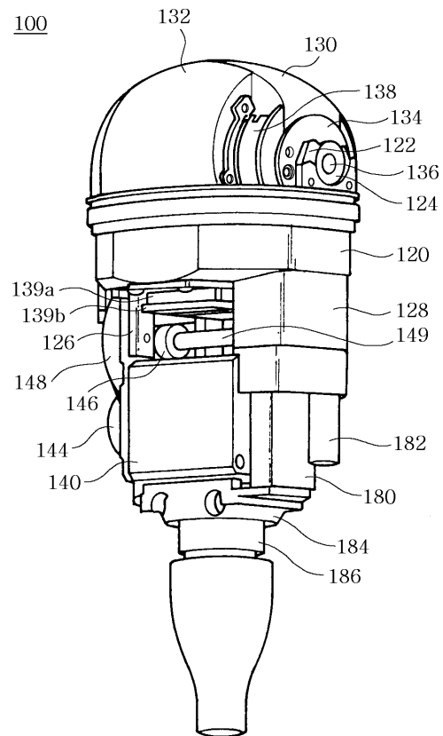
도면3
