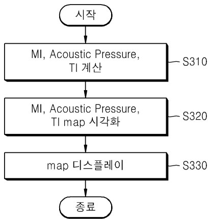
도면4
