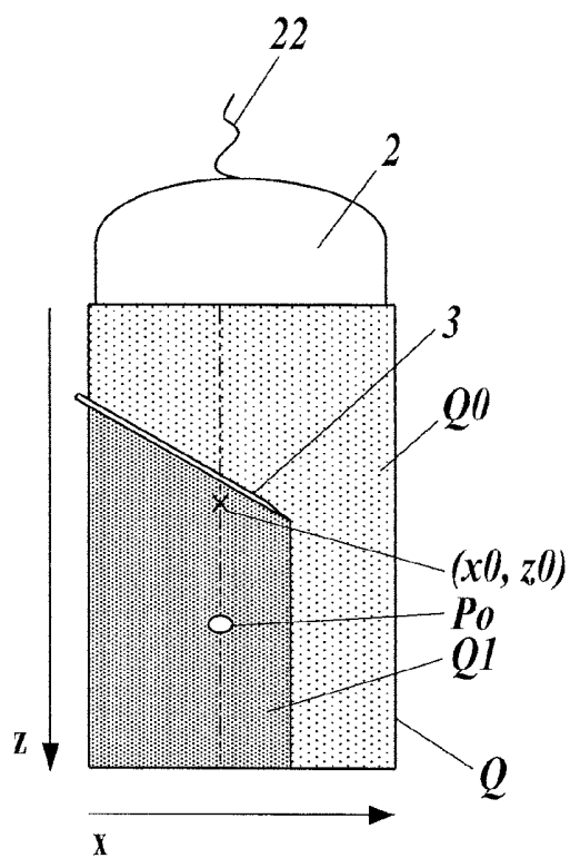
FIG.13A
