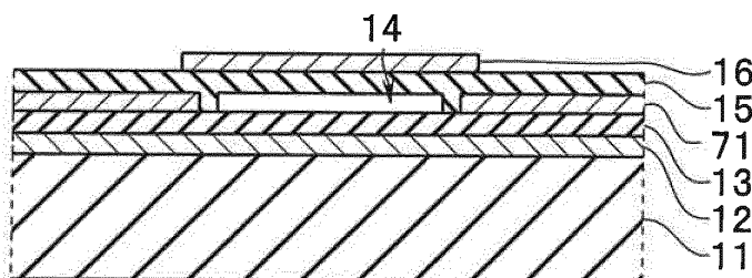
FIG.13E
