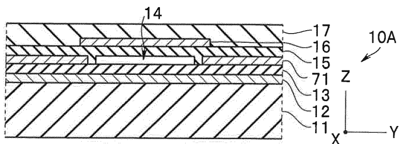
FIG.13F
