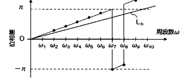
(b) 一部位相修正を行った状態
