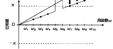
(d) 過度に位相修正を行った状態
