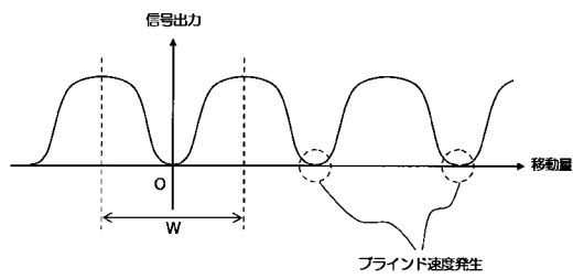
(a) 従来のノリスドブラ法におけるMTIフィルタ
