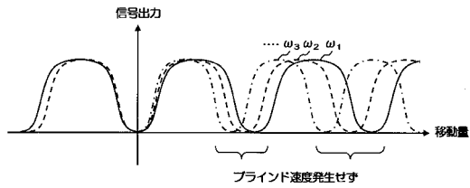
(b) 広帯域ドブラ法におけるMTIフィルタ
