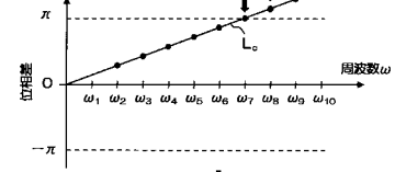
(c) 適正に位相修正を行った状態
