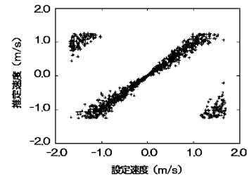
(c) 本発明に係る広帯域ドブラ法
