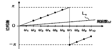
(a) 位相修正を行っていない状態
