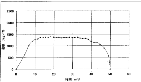
位置／速度併用制御方式における速度特性例
