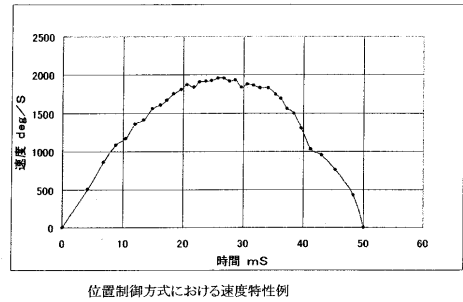
位置制御方式における速度特性例
