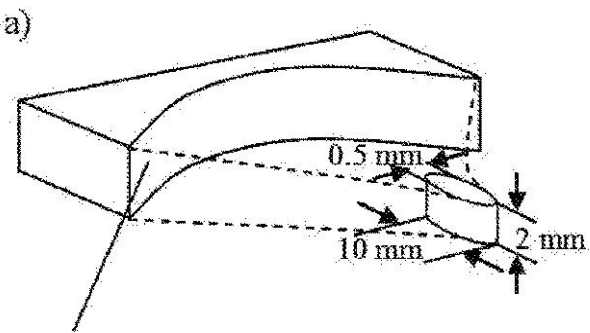
広開口円筒形単一要素 トランスデューサー、 f = 100 \text{ mm}
