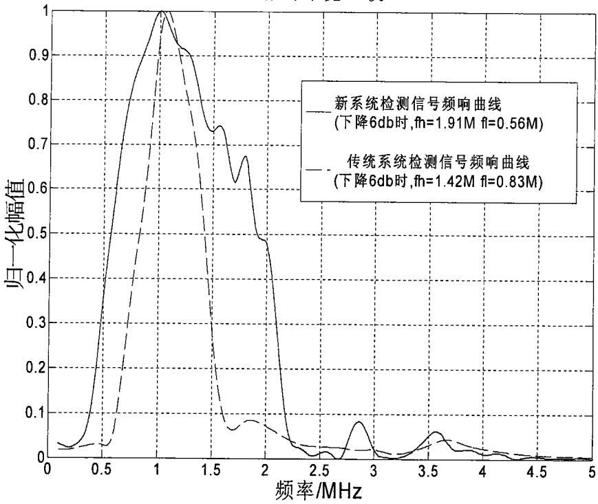
图 5c 相对带宽比较
