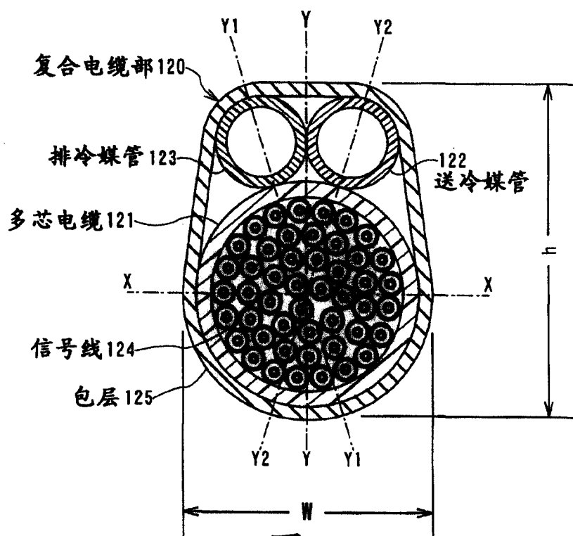
图 30 现有技术
