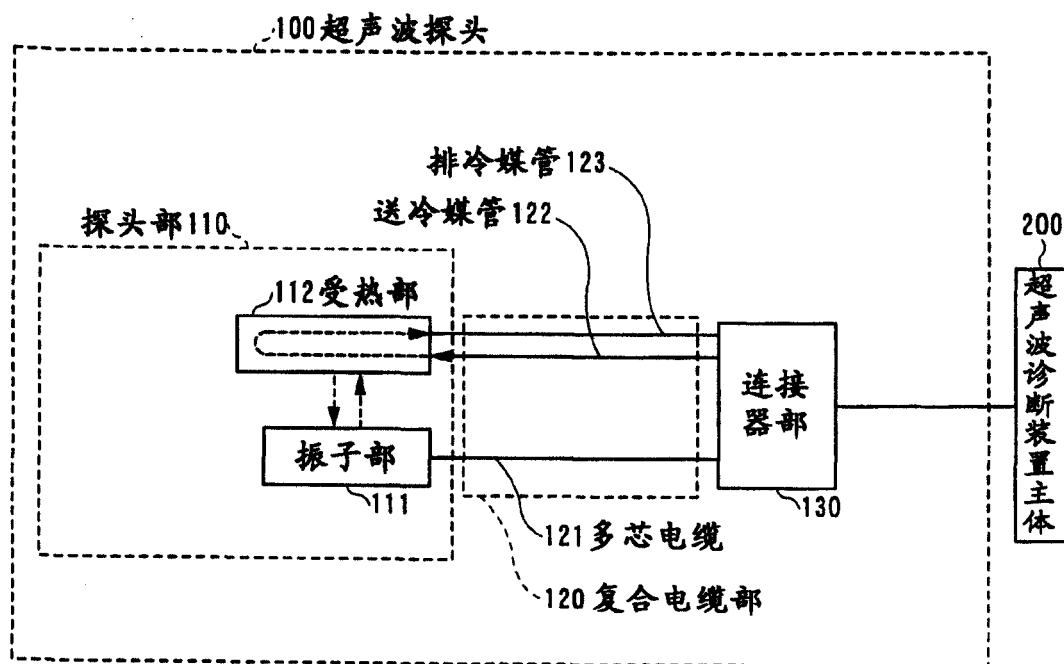
图 29 现有技术
