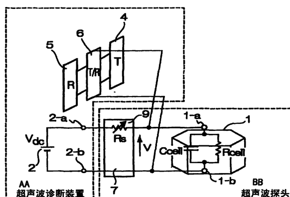
AA— 超声波诊断装置 BB— 超声波探头
