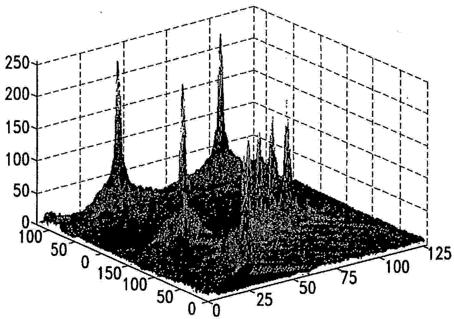
图6中放大区域的透视图，图像点处于 1/2 的波长间隔。 粉红色表示处于 -48\text{DB} 或更低的旁瓣，且深蓝色表示 低于 -100\text{DB} 的背景杂斑。 沿X轴和Y轴的刻度以 1/2 个波长为单位。
