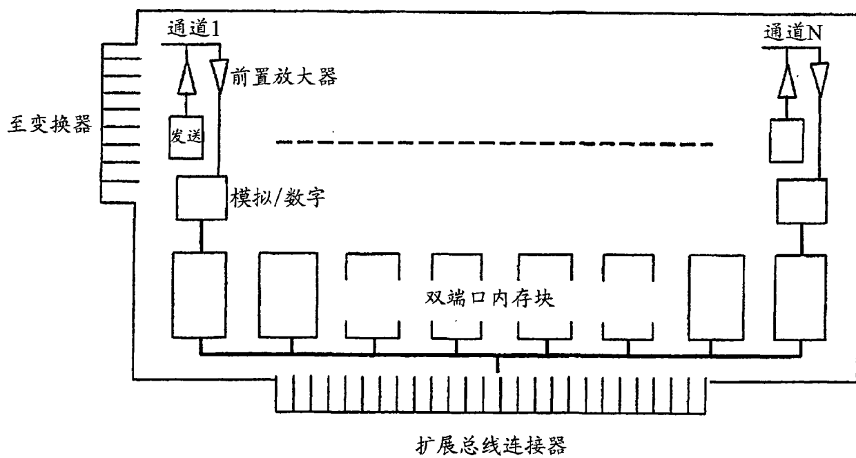
包含采集电路的插件模块的示意图
