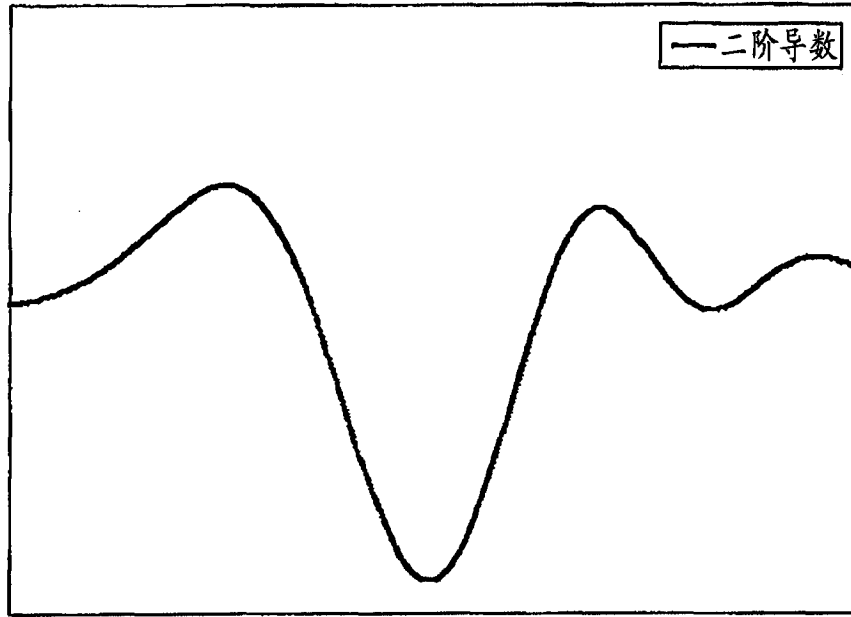
二阶导数
