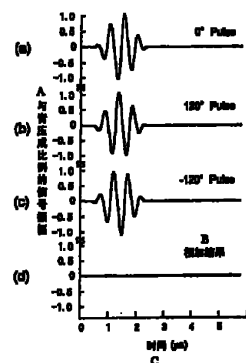
A 与背压成比例的信号振幅 B 相加結果 C 时间
