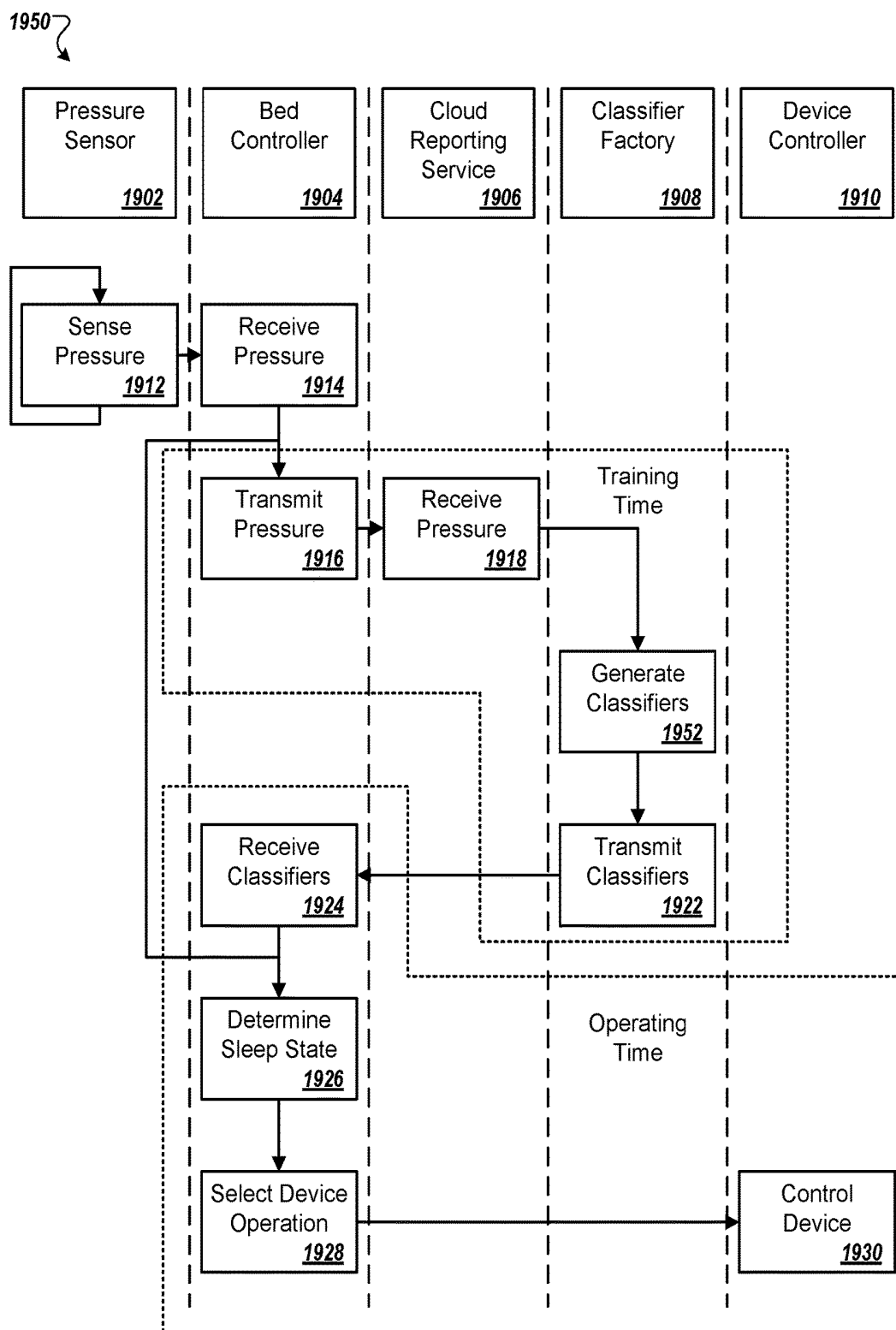
FIG. 19B
