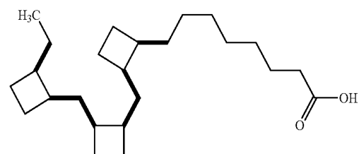
8-{2-[2-(2-Ethyl-cyclobutylmethyl)-cyclobutylmethyl]-cyclobutyl}-octanoic acid
