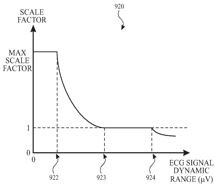
FIG. 9C
