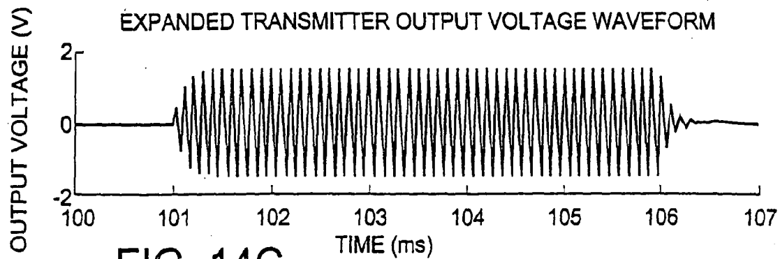
FIG. 14C.
